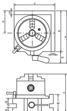
5C COLLET INDEXER NON ECONOMICAL
