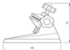
MICROMETER STAND
